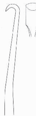
CS-3549-02 23 cm / 9" 9 mm Right rechts droit derecho
